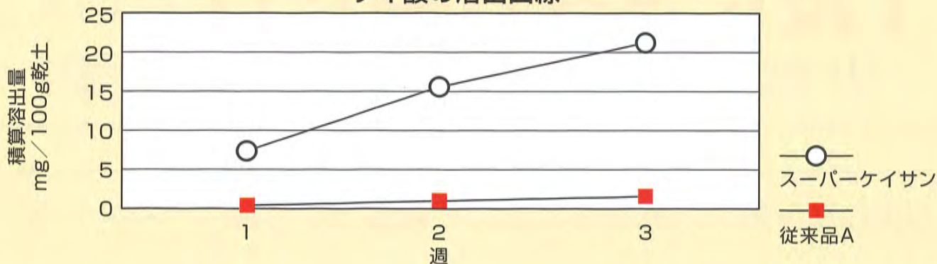
ケイ酸の溶出曲線
